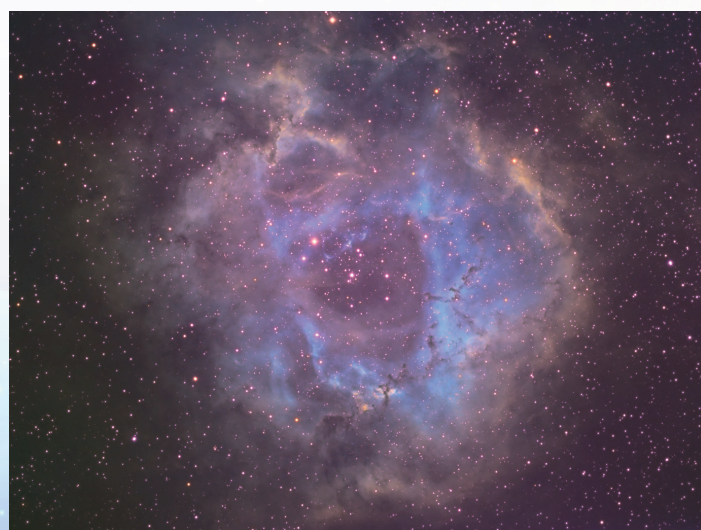
NGC 2244 (麒麟座玫瑰星雲 SHO版)
